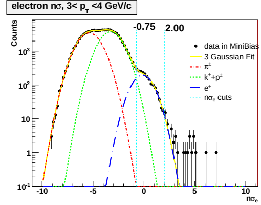
(b) MinBias 3 < p_T < 4 GeV/c
