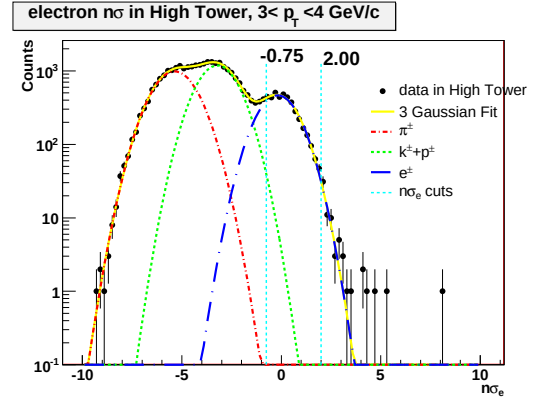
(d) High Tower 3 < p_T < 4 GeV/c
