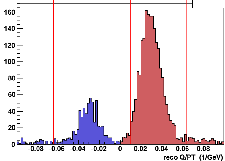
reco Q/PT,W ET>25 GeV
