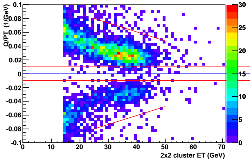
TPC PRIM Q/PT
