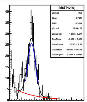
mom-slice-6.5&lt;P&lt;7.0
