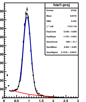
mom-slice-5.0&lt;P&lt;5.5
