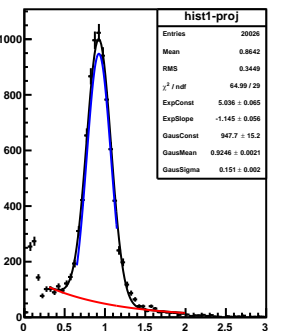
mom-slice-5.5&lt;P&lt;6.0
