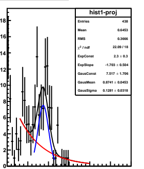
mom-slice-7.5&lt;P&lt;8.0
