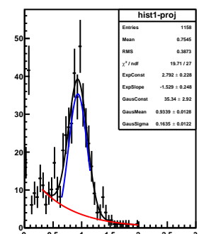
mom-slice-8.5&lt;P&lt;9.0
