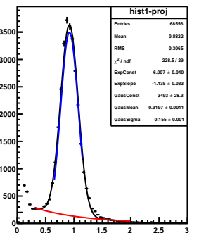
mom-slice-4.5&lt;P&lt;5.0
