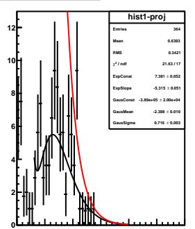
mom-slice-8.0&lt;P&lt;8.5
