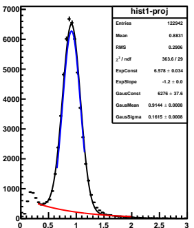
mom-slice-4.0&lt;P&lt;4.5
