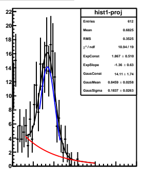
mom-slice-7.0&lt;P&lt;7.5
