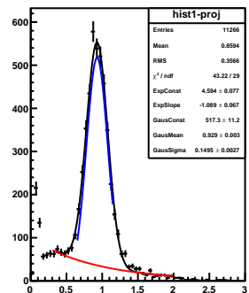
mom-slice-6.0&lt;P&lt;6.5
