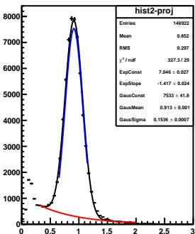
mom-slice-4.5&lt;P&lt;5.0
