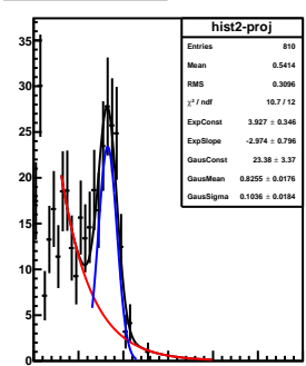
mom-slice-6.5&lt;P&lt;7.0
