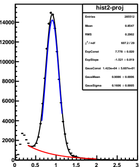
mom-slice-4.0&lt;P&lt;4.5
