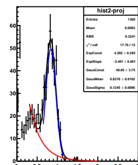
mom-slice-8.5&lt;P&lt;9.0
