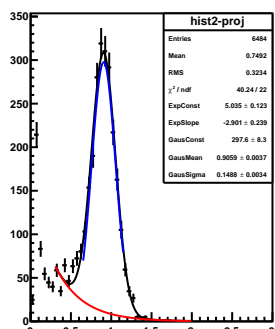
mom-slice-7.0&lt;P&lt;7.5
