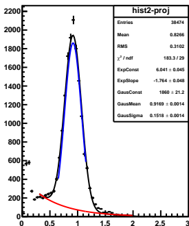
mom-slice-5.5&lt;P&lt;6.0
