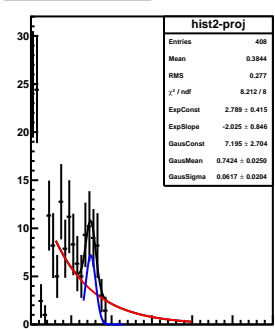
mom-slice-7.5&lt;P&lt;8.0
