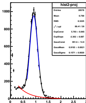
mom-slice-6.0&lt;P&lt;6.5
