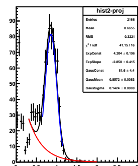
mom-slice-8.0&lt;P&lt;8.5
