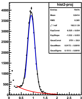
mom-slice-5.0&lt;P&lt;5.5
