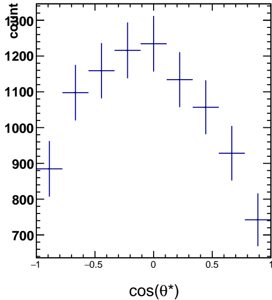
RawYields 2.4 < p_T < 3.0 , 3\pi/6 < \phi^* < 4\pi/6
