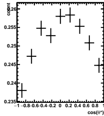
Efficiency 0/5 < y < 1/5 , 7\pi/6 < \phi' < 8\pi/6
