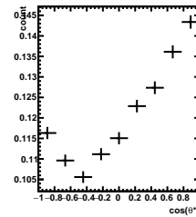
Efficiency -4/5 < y < -3/5 , 4\pi/6 < \phi' < 5\pi/6
