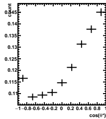
Efficiency -4/5 < y < -3/5 , 7\pi/6 < \phi' < 8\pi/6
