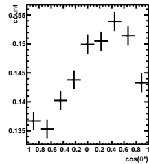
Efficiency -4/5 < y < -3/5, 3\pi/6 < \phi' < 4\pi/6
