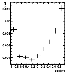
Efficiency -5/5 < y < -4/5 , 7\pi/6 < \phi' < 8\pi/6
