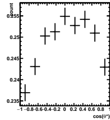
Efficiency 0/5 < y < 1/5, 3\pi/6 < \phi' < 4\pi/6
