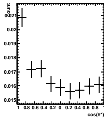
Efficiency -5/5 < y < -4/5 , 2\pi/6 < \phi' < 3\pi/6
