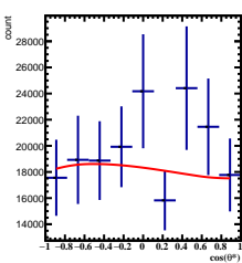
Corrected Yields -4/5 < y < -3/5 , 3\pi/6 < \phi < 4\pi/6
