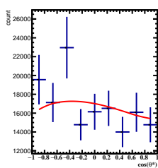
Corrected Yields -1/5 < y < 0/5 , 3\pi/6 < \phi < 4\pi/6
