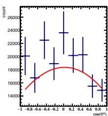
Corrected Yields 0/5 < y < 1/5 , 3\pi/6 < \phi < 4\pi/6
