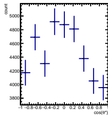
RawYields -3/5 < y < -2/5 , 8\pi/6 < \psi' < 9\pi/6
