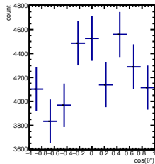
RawYields -3/5 < y < -2/5 , 4\pi/6 < \phi' < 5\pi/6
