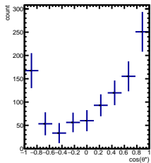
RawYields -5/5 < y < -4/5 , 4\pi/6 < \phi' < 5\pi/6
