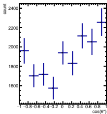
RawYields -4/5 < y < -3/5 , 4\pi/6 < \phi' < 5\pi/6
