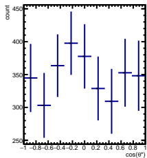
RawYields -5/5 < y < -4/5 , 3\pi/6 < \phi' < 4\pi/6
