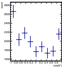
RawYields -4/5 < y < -3/5 , 1\pi/6 < \phi' < 2\pi/6
