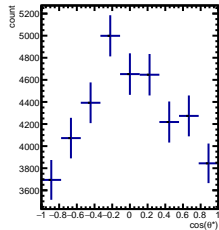
RawYields 2/5 < y < 3/5 , 2\pi/6 < \phi' < 3\pi/6
