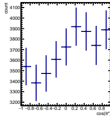
RawYields -3/5 < y < -2/5 , 6\pi/6 < \phi' < 7\pi/6
