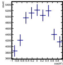
RawYields -2/5 < y < -1/5 , 2\pi/6 < \phi' < 3\pi/6
