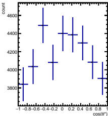
RawYields 1/5 < y < 2/5 , 7\pi/6 < \phi < 8\pi/6
