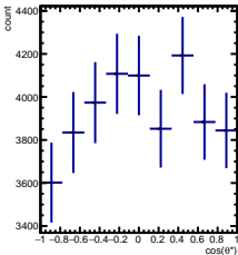
RawYields 2/5 < y < 3/5 , 7\pi/6 < \phi < 8\pi/6
