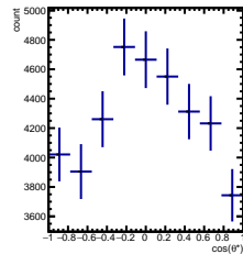
RawYields -1/5 < y < 0/5 , 4\pi/6 < \phi' < 5\pi/6
