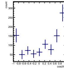
RawYields 4/5 < y < 5/5 , 10\pi/6 < \phi < 11\pi/6
