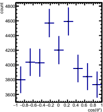
RawYields 0/5 < y < 1/5 , 7\pi/6 < \phi < 8\pi/6
