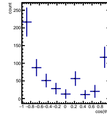
RawYields 4/5 < y < 5/5 , 6\pi/6 < \phi' < 7\pi/6
