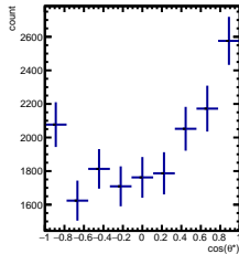
RawYields 3/5 < y < 4/5 , 10\pi/6 < \phi < 11\pi/6
