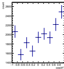
RawYields 3/5 < y < 4/5 , 1\pi/6 < \phi' < 2\pi/6
