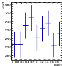
RawYields 3/5 < y < 4/5 , 8\pi/6 < \psi' < 9\pi/6
