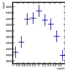
RawYields -2/5 < y < -1/5 , 3\pi/6 < \phi' < 4\pi/6
