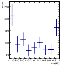
RawYields -5/5 < y < -4/5 , 10\pi/6 < \phi < 11\pi/6
