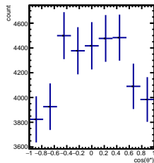
RawYields 2/5 < y < 3/5 , 8\pi/6 < \psi' < 9\pi/6
