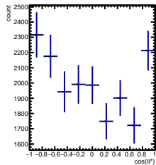
RawYields 3/5 < y < 4/5 , 4\pi/6 < \phi' < 5\pi/6
