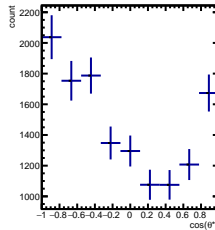
RawYields 3/5 < y < 4/5 , 6\pi/6 < \phi' < 7\pi/6
