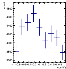
RawYields -1/5 < y < 0/5 , 5\pi/6 < \phi' < 6\pi/6
