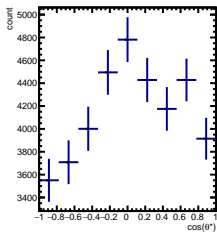
RawYields 1/5 < y < 2/5 , 4\pi/6 < \phi' < 5\pi/6
