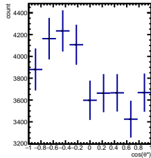
RawYields -3/5 < y < -2/5 , 11\pi/6 < \phi' < 12\pi/6
