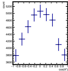
RawYields -1/5 < y < 0/5 , 2\pi/6 < \phi' < 3\pi/6
