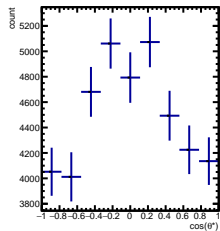
RawYields -2/5 < y < -1/5 , 4\pi/6 < \phi' < 5\pi/6
