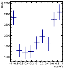
RawYields -4/5 < y < -3/5 , 7\pi/6 < \phi < 8\pi/6
