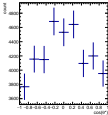
RawYields 1/5 < y < 2/5 , 10\pi/6 < \phi < 11\pi/6
