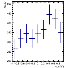
RawYields 4/5 < y < 5/5 , 2\pi/6 < \phi' < 3\pi/6
