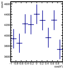
RawYields -3/5 < y < -2/5 , 7\pi/6 < \phi < 8\pi/6
