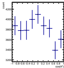
RawYields 2/5 < y < 3/5 , 4\pi/6 < \phi' < 5\pi/6
