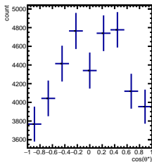
RawYields 1/5 < y < 2/5 , 8\pi/6 < \psi' < 9\pi/6
