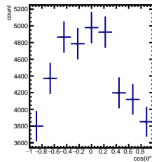
RawYields -1/5 < y < 0/5 , 3\pi/6 < \phi' < 4\pi/6
