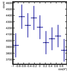
RawYields -3/5 < y < -2/5 , 10\pi/6 < \phi < 11\pi/6
