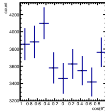
RawYields 2/5 < y < 3/5 , 6\pi/6 < \phi' < 7\pi/6
