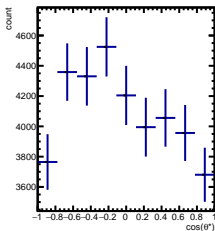
RawYields 0/5 < y < 1/5 , 5\pi/6 < \phi' < 6\pi/6
