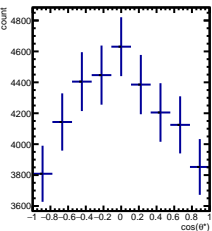
RawYields 0/5 < y < 1/5 , 1\pi/6 < \phi' < 2\pi/6
