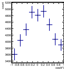
RawYields 1/5 < y < 2/5 , 3\pi/6 < \phi' < 4\pi/6
