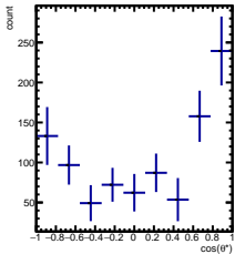
RawYields -5/5 < y < -4/5 , 7\pi/6 < \phi < 8\pi/6
