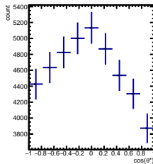
RawYields -2/5 < y < -1/5 , 1\pi/6 < \phi' < 2\pi/6
