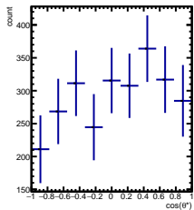
RawYields -5/5 < y < -4/5 , 8\pi/6 < \psi' < 9\pi/6
