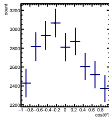
RawYields 3/5 < y < 4/5 , 3\pi/6 < \phi' < 4\pi/6
