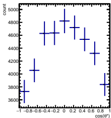
RawYields 0/5 < y < 1/5 , 3\pi/6 < \phi' < 4\pi/6
