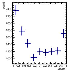
RawYields 3/5 < y < 4/5 , 5\pi/6 < \phi' < 6\pi/6
