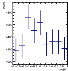
RawYields -2/5 < y < -1/5 , 5\pi/6 < \phi' < 6\pi/6
