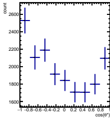
RawYields -4/5 < y < -3/5 , 10\pi/6 < \phi < 11\pi/6
