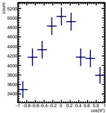
RawYields 0/5 < y < 1/5 , 2\pi/6 < \phi' < 3\pi/6
