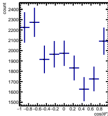
RawYields 3/5 < y < 4/5 , 7\pi/6 < \phi < 8\pi/6
