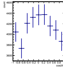
RawYields -1/5 < y < 0/5 , 6\pi/6 < \phi' < 7\pi/6
