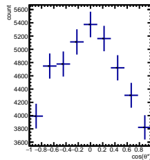
RawYields -3/5 < y < -2/5 , 3\pi/6 < \phi' < 4\pi/6
