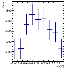
RawYields -2/5 < y < -1/5 , 10\pi/6 < \phi < 11\pi/6
