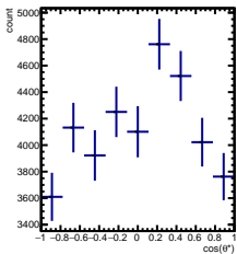
RawYields 0/5 < y < 1/5 , 4\pi/6 < \phi' < 5\pi/6
