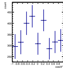
RawYields 4/5 < y < 5/5 , 3\pi/6 < \phi' < 4\pi/6
