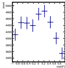
RawYields -1/5 < y < 0/5 , 8\pi/6 < \psi' < 9\pi/6
