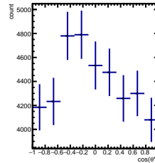
RawYields -2/5 < y < -1/5 , 11\pi/6 < \phi' < 12\pi/6
