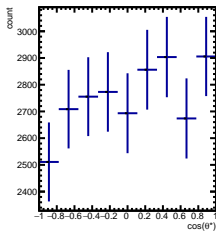
RawYields -4/5 < y < -3/5 , 8\pi/6 < \psi' < 9\pi/6
