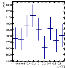
RawYields 2/5 < y < 3/5 , 10\pi/6 < \phi < 11\pi/6
