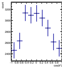
RawYields -4/5 < y < -3/5 , 3\pi/6 < \phi' < 4\pi/6
