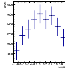
RawYields -1/5 < y < 0/5 , 10\pi/6 < \phi < 11\pi/6
