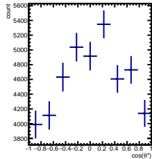
RawYields -3/5 < y < -2/5 , 2\pi/6 < \phi' < 3\pi/6
