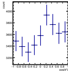
RawYields 2/5 < y < 3/5 , 11\pi/6 < \phi' < 12\pi/6
