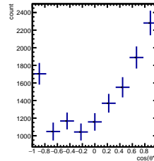
RawYields 3/5 < y < 4/5 , 11\pi/6 < \phi' < 12\pi/6
