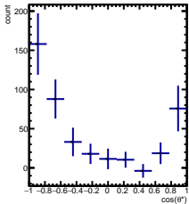
RawYields -5/5 < y < -4/5 , 11\pi/6 < \phi' < 12\pi/6
