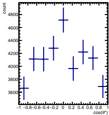
RawYields 0/5 < y < 1/5 , 10\pi/6 < \phi < 11\pi/6
