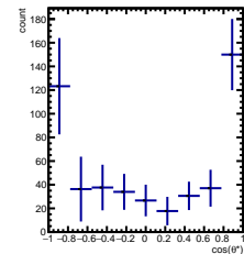
RawYields 4/5 < y < 5/5 , 5\pi/6 < \phi' < 6\pi/6
