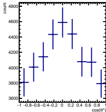
RawYields 1/5 < y < 2/5 , 11\pi/6 < \phi' < 12\pi/6
