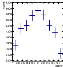
RawYields 2/5 < y < 3/5 , 3\pi/6 < \phi' < 4\pi/6
