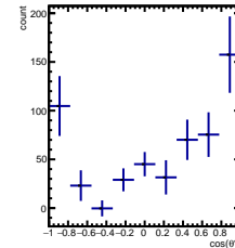
RawYields 4/5 < y < 5/5 , 11\pi/6 < \phi' < 12\pi/6
