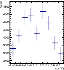
RawYields 0/5 < y < 1/5 , 9\pi/6 < \phi' < 10\pi/6
