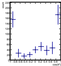
RawYields -5/5 < y < -4/5 , 5\pi/6 < \phi' < 6\pi/6
