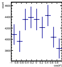
RawYields -1/5 < y < 0/5 , 1\pi/6 < \phi' < 2\pi/6
