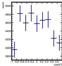
RawYields -2/5 < y < -1/5 , 8\pi/6 < \psi' < 9\pi/6
