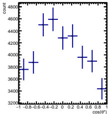
RawYields 0/5 < y < 1/5 , 11\pi/6 < \phi' < 12\pi/6
