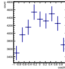
RawYields -1/5 < y < 0/5 , 11\pi/6 < \phi' < 12\pi/6
