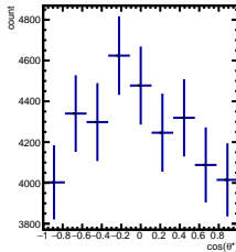
RawYields -1/5 < y < 0/5 , 7\pi/6 < \phi < 8\pi/6
