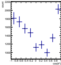
RawYields -4/5 < y < -3/5 , 11\pi/6 < \phi' < 12\pi/6
