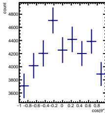
RawYields 1/5 < y < 2/5 , 6\pi/6 < \phi' < 7\pi/6
