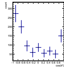
RawYields 4/5 < y < 5/5 , 4\pi/6 < \phi' < 5\pi/6
