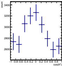
RawYields -4/5 < y < -3/5 , 2\pi/6 < \phi' < 3\pi/6
