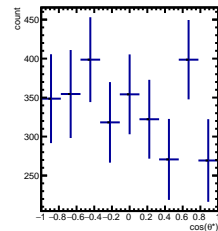
RawYields 4/5 < y < 5/5 , 8\pi/6 < \psi' < 9\pi/6
