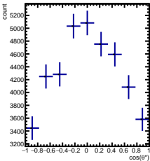
RawYields 1/5 < y < 2/5 , 2\pi/6 < \phi' < 3\pi/6
