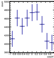
RawYields -2/5 < y < -1/5 , 7\pi/6 < \phi < 8\pi/6
