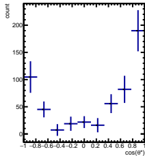
RawYields -5/5 < y < -4/5 , 6\pi/6 < \phi' < 7\pi/6
