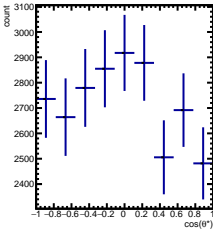
RawYields -4/5 < y < -3/5 , 9\pi/6 < \phi' < 10\pi/6
