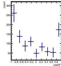
RawYields 4/5 < y < 5/5 , 7\pi/6 < \phi < 8\pi/6
