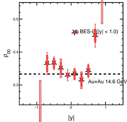
1.00 &lt;math&gt;p_T&lt;/math&gt; &lt; 2.00 GeV/c, Cent (0-10)
