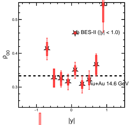
2.00 &lt;math&gt;p_T&lt;/math&gt; &lt; 5.00 GeV/c, Cent (10-40)
