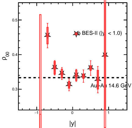
1.00 &lt;math&gt;p_T&lt;/math&gt; &lt; 2.00 GeV/c, Cent (40-80)
