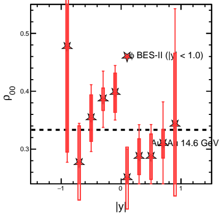
2.00 &lt;math&gt;p_T&lt;/math&gt; &lt; 5.00 GeV/c, Cent (40-80)
