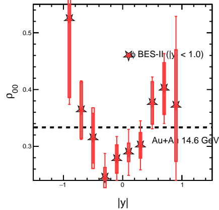
2.00 &lt;math&gt;p_T&lt;/math&gt; &lt; 5.00 GeV/c, Cent (0-10)
