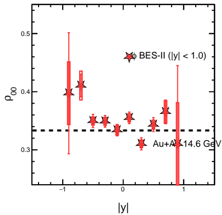
1.00 &lt;math&gt;p_T&lt;/math&gt; &lt; 2.00 GeV/c, Cent (10-40)
