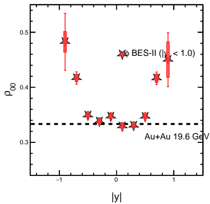
1.00 <math>p_T</math> <math>< 2.00</math> GeV/c, Cent (10-40)
