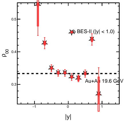
1.00 <math>p_T</math> <math>< 2.00</math> GeV/c, Cent (40-80)
