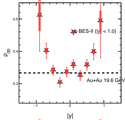
1.00 <math>p_T</math> <math>< 2.00</math> GeV/c, Cent (0-10)
