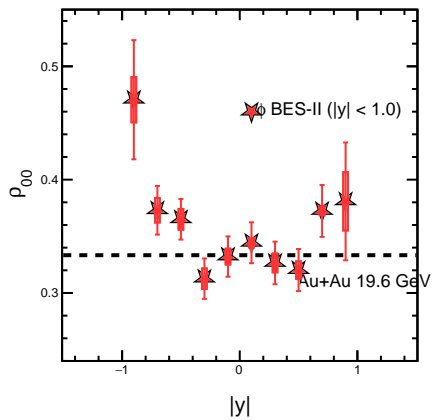
2.00 <math>p_T</math> <math>< 5.00</math> GeV/c, Cent (10-40)
