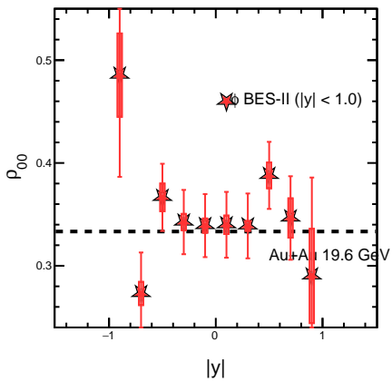
2.00 <math>p_T</math> <math>< 5.00</math> GeV/c, Cent (40-80)
