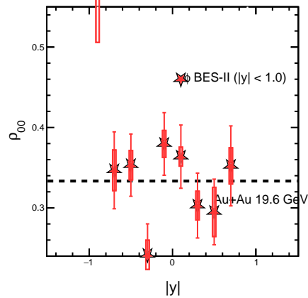
2.00 <math>p_T</math> <math>< 5.00</math> GeV/c, Cent (0-10)
