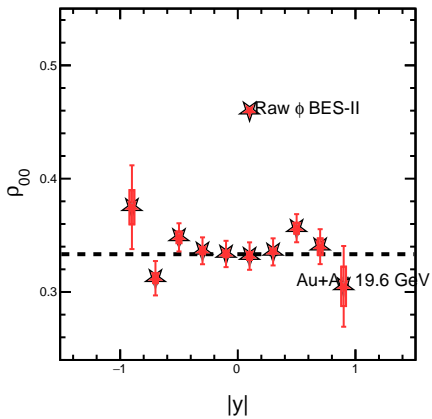
2.00 &lt;math&gt;p_T&lt;/math&gt; &lt;math&gt;&lt; 5.00&lt;/math&gt; GeV/c, Cent (40-80)
