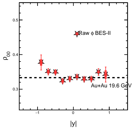
2.00 &lt;math&gt;p_T&lt;/math&gt; &lt;math&gt;&lt; 5.00&lt;/math&gt; GeV/c, Cent (10-40)
