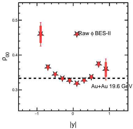
1.00 &lt;math&gt;p_T&lt;/math&gt; &lt;math&gt;&lt; 2.00&lt;/math&gt; GeV/c, Cent (40-80)
