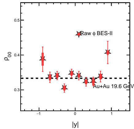
2.00 &lt;math&gt;p_T&lt;/math&gt; &lt;math&gt;&lt; 5.00&lt;/math&gt; GeV/c, Cent (0-10)
