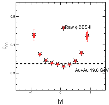
1.00 &lt;math&gt;p_T&lt;/math&gt; &lt;math&gt;&lt; 2.00&lt;/math&gt; GeV/c, Cent (10-40)
