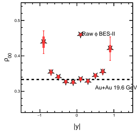
1.00 &lt;math&gt;p_T&lt;/math&gt; &lt;math&gt;&lt; 2.00&lt;/math&gt; GeV/c, Cent (0-10)
