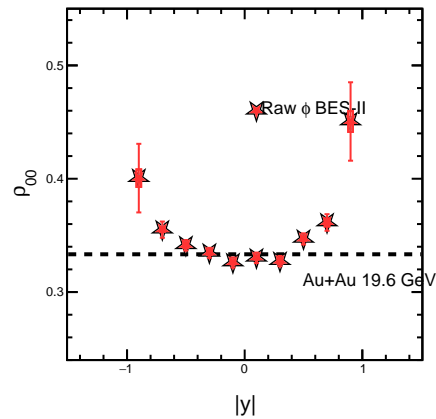
1.00 &lt;math&gt;p_T &lt; 2.00 &lt;/math&gt; GeV/c, Cent (0-10)
