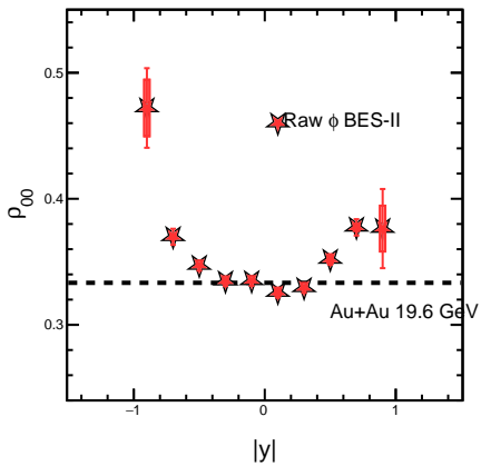
1.00 &lt;math&gt;p_T &lt; 2.00 &lt;/math&gt; GeV/c, Cent (40-80)
