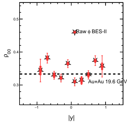
2.00 &lt;math&gt;p_T &lt; 5.00 &lt;/math&gt; GeV/c, Cent (0-10)
