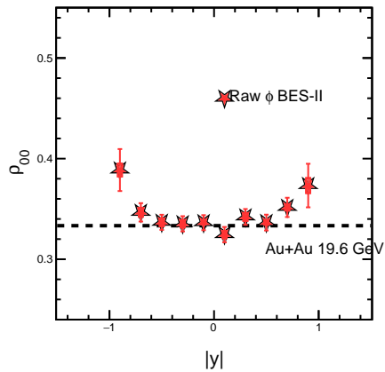
2.00 &lt;math&gt;p_T &lt; 5.00 &lt;/math&gt; GeV/c, Cent (10-40)
