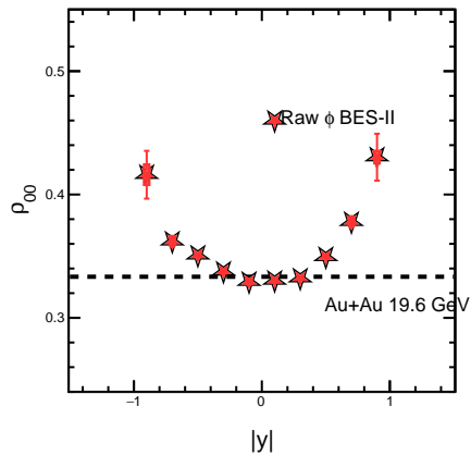
1.00 &lt;math&gt;p_T &lt; 2.00 &lt;/math&gt; GeV/c, Cent (10-40)
