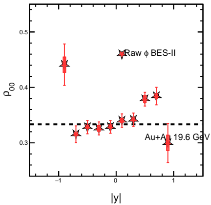
2.00 &lt;math&gt;p_T &lt; 5.00 &lt;/math&gt; GeV/c, Cent (40-80)
