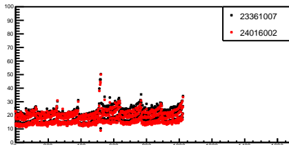
g_totStdDev_11_2
