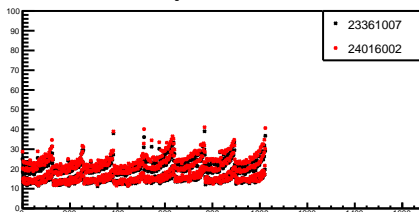
g_totStdDev_23_1
