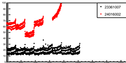
g_totStdDev_35_2
