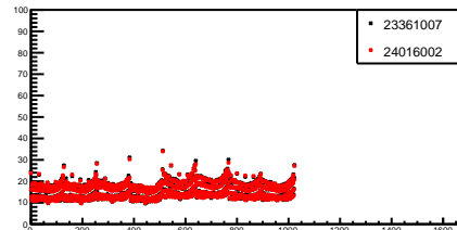
g_ranStdDev_2_1
