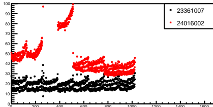
g_totStdDev_25_2
