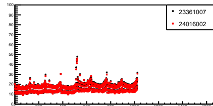
g_ranStdDev_11_1
