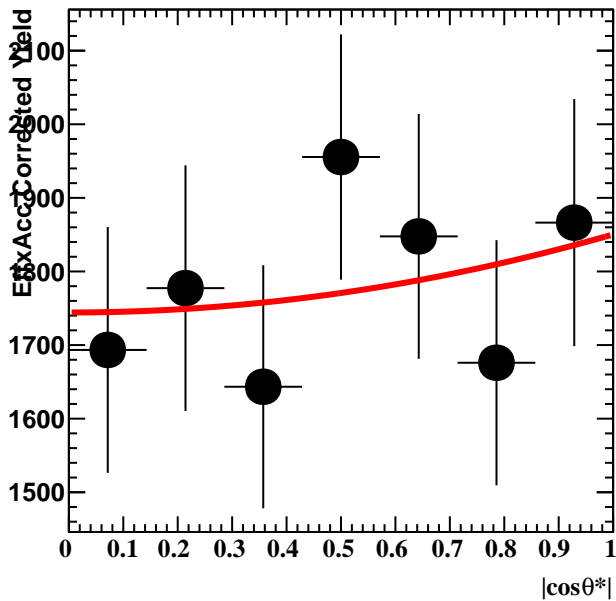
3.0 <math>p_T</math> <math>< 4.2\text{ GeV}/c</math>, Cent 20-60
