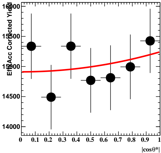
2.4 <math>p_T</math> <math>< 3.0\text{ GeV}/c</math>, Cent 20-60
