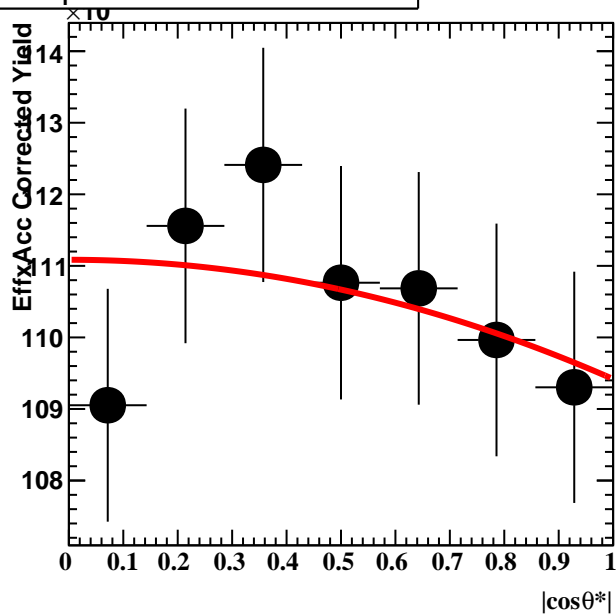
1.8 <math>p_T</math> <math>< 2.4\text{ GeV}/c</math>, Cent 20-60
