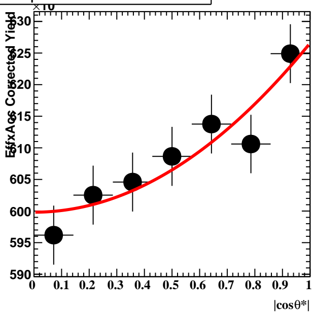
1.2 <math>p_T</math> <math>< 1.8\text{ GeV}/c</math>, Cent 20-60
