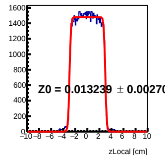
Module 6 Tray26 : z Local Fit
