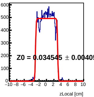
Module 4 Tray55 : z Local Fit
