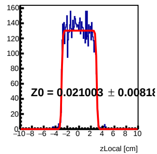
Module 2 Tray82 : z Local Fit
