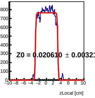
Module 0 Tray62 : z Local Fit
