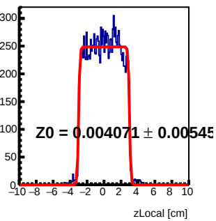
Module 1 Tray55 : z Local Fit
