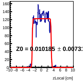
Module 2 Tray16 : z Local Fit
