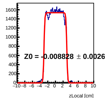
Module 6 Tray14 : z Local Fit
