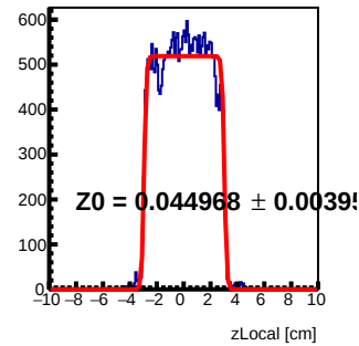
Module 4 Tray83 : z Local Fit
