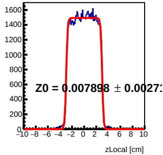
Module 6 Tray40 : z Local Fit
