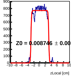
Module 0 Tray63 : z Local Fit
