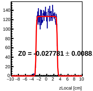
Module 2 Tray12 : z Local Fit
