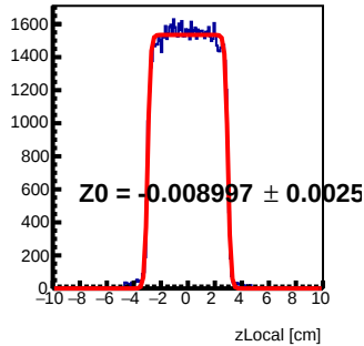
Module 6 Tray28 : z Local Fit
