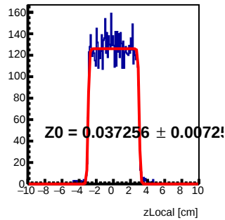
Module 2 Tray21 : z Local Fit
