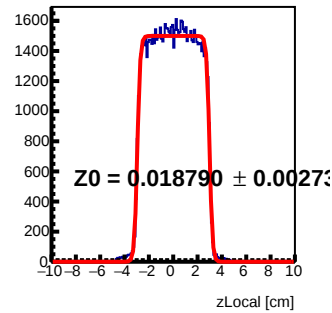
Module 6 Tray46 : z Local Fit
