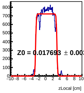
Module 0 Tray61 : z Local Fit
