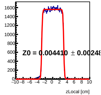
Module 6 Tray34 : z Local Fit
