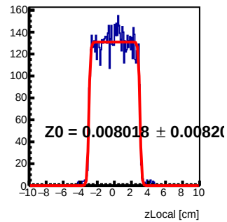
Module 2 Tray78 : z Local Fit
