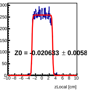
Module 1 Tray59 : z Local Fit
