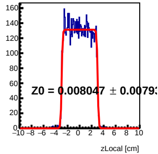
Module 2 Tray9 : z Local Fit
