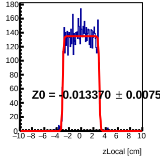
Module 2 Tray17 : z Local Fit
