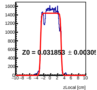
Module 6 Tray10 : z Local Fit
