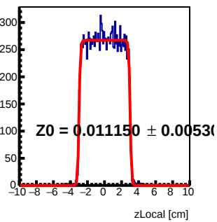
Module 1 Tray47 : z Local Fit
