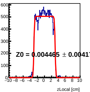
Module 4 Tray63 : z Local Fit
