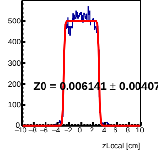
Module 4 Tray71 : z Local Fit
