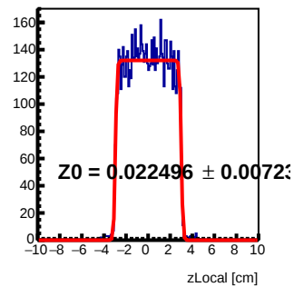
Module 2 Tray74 : z Local Fit
