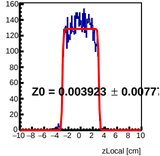
Module 2 Tray13 : z Local Fit
