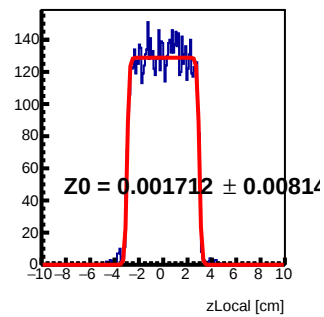
Module 2 Tray70 : z Local Fit
