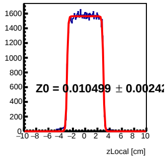
Module 6 Tray44 : z Local Fit
