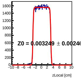
Module 6 Tray32 : z Local Fit
