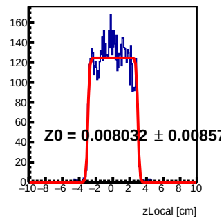
Module 2 Tray66 : z Local Fit
