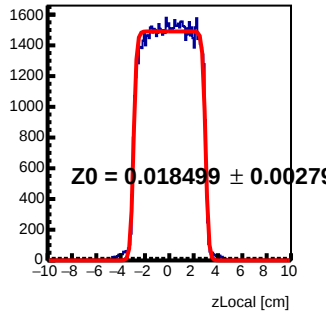
Module 6 Tray36 : z Local Fit
